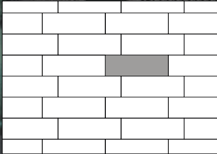
Verlegemuster: 1/4 Verband, 90 x 30 x 4 cm
